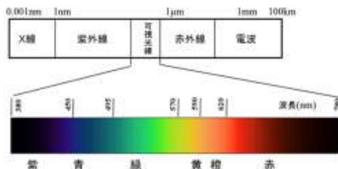
図 1 - 6 : 光の波長
