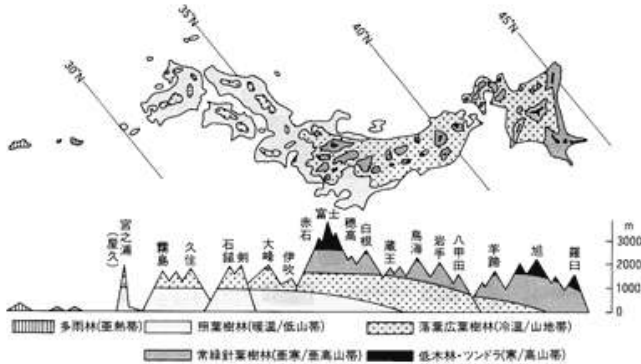
図 3-3 : 日本のバイオームの水平・垂直分布
